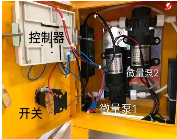
内部结构图
